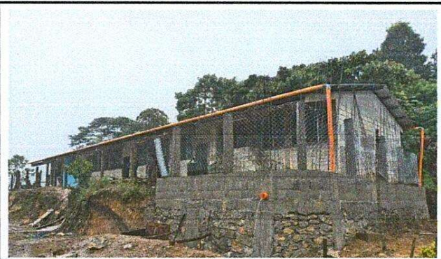
Foto 2: RESULTADOS FINAL DE CIMIENTA DE MURO DE CONTENCIÓN PARA REFORZAR LOS COLUMNAS DE MALLAS Y TAMBIEN EL EDIFICIOS ESCOLAR.
